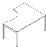
BOY10 1600 / 1200 / 740 45,6 kg
