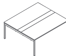
SY08 1800 / 1610 / 740 88.5 kg
