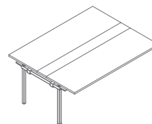
SY38 1800 / 1410 / 740 67.4 kg
