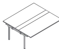
SY18 1800 / 1610 / 740 80.3 kg
