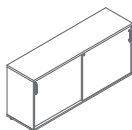
A3P16 1610 / 432 / 1129 68 kg
